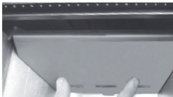
Fig. 14: soulever la plaque coupe-flamme
